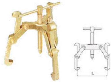
NS273 3 Leg Gear Puller
